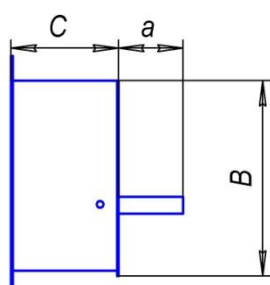
Рис.3. Размеры вылета заслонки в открытом положении за пределы корпуса клапана исп. 60-КИД, 60-КИД(МС).
