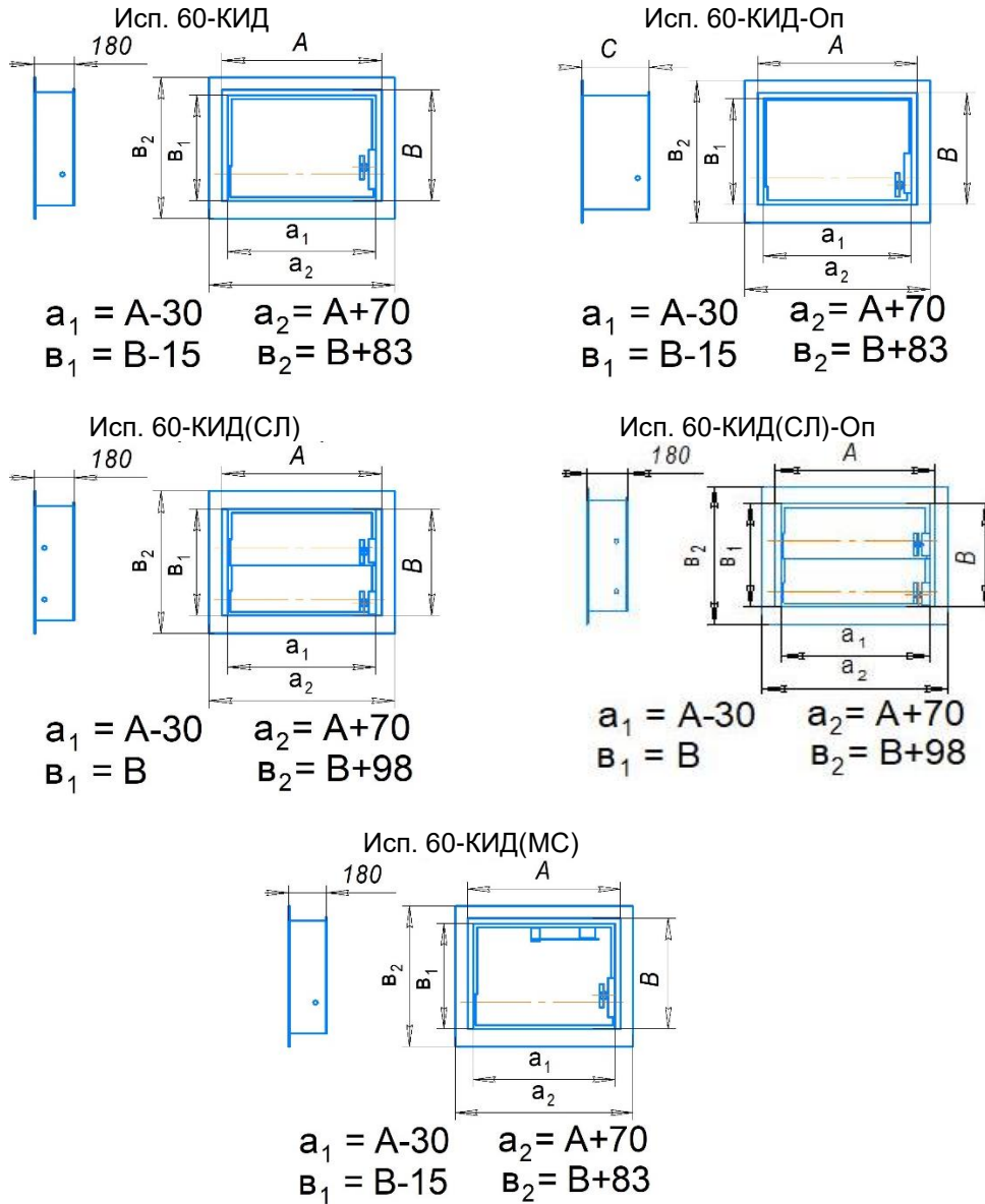
Рис.1. Установочные (A, B), внутреннего сечения (a 1 , b 1 ) и габаритные (a 2 , b 2 ) размеры «стенового» клапана.
