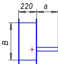
Рис.3а. Размеры вылета заслонки в открытом положении за пределы корпуса клапана исп. 60-КИД-Оп.
