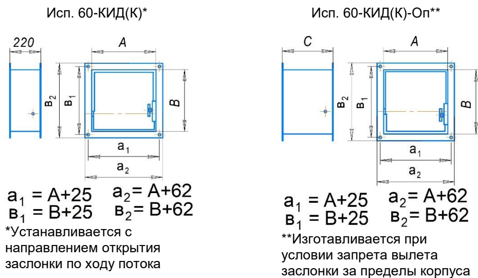
Рис.1а. Внутреннего размера (A, B), установочные (a 1 , b 1 ) и габаритные (a 2 , b 2 ) размеры «канального» клапана.
